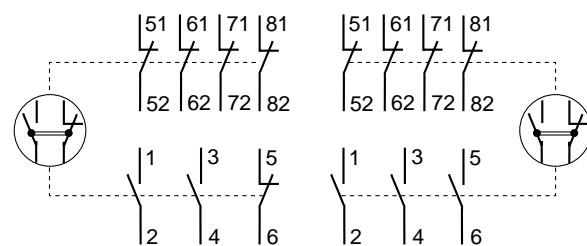
104S-C30⊗008C...C85⊗008C
